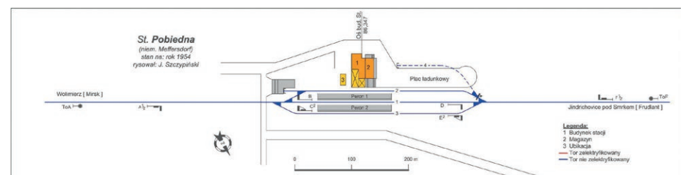
Szkic stacji Pobiedna rys. J. Szczypiński (stan na 1954 rok)
