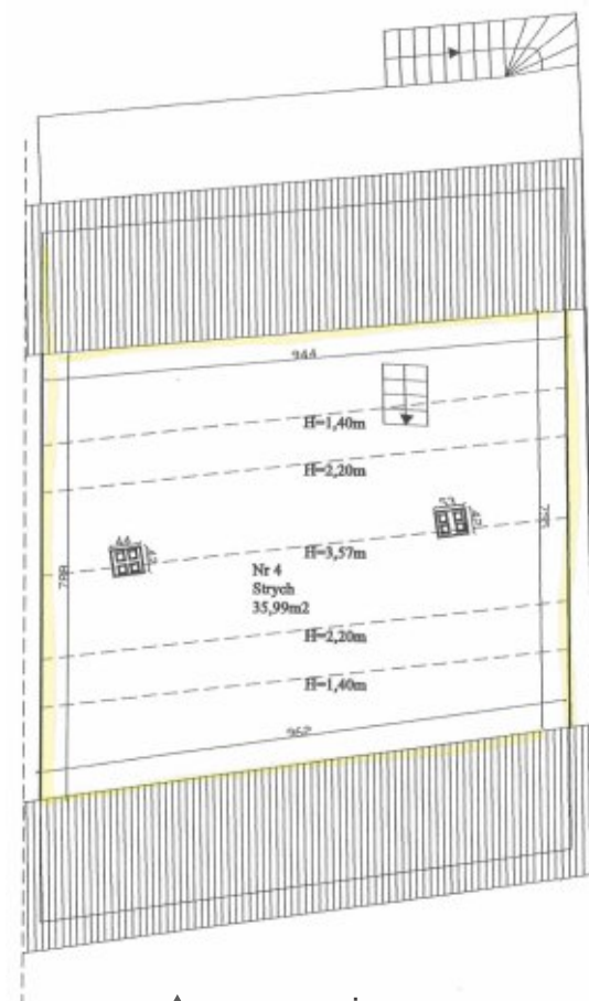
▲ Leśna, ul. Żeromskiego nr 7 budynek mieszkalno-usługowy rzut strychu wys 3,57m
