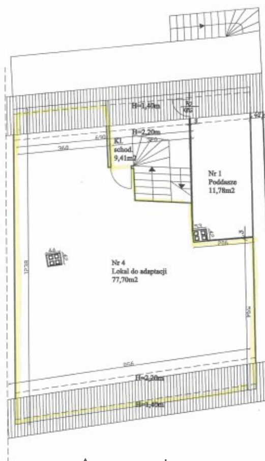
▲ Leśna, ul. Żeromskiego nr 7 budynek mieszkalno-usługowy rzut poddasza wys 2,95m
